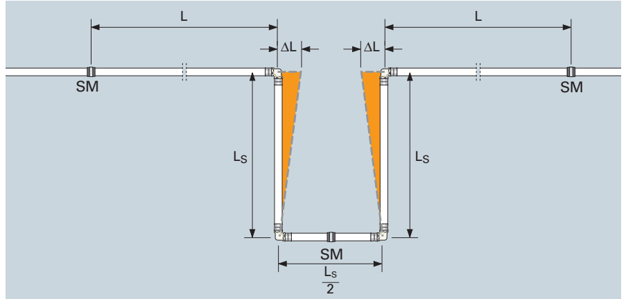
Boyca genleşmenin bir "omega" ile dengelenmesi
