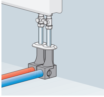
Radyatör bağlantı dirseğiyle kolektörden alpex tekli bağlantı
