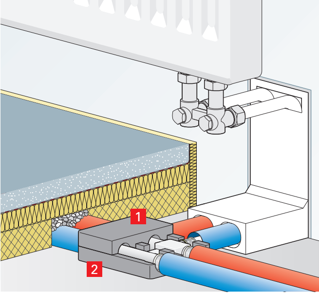
1 Sap katmanında ses köprüsünün engellenmesi
