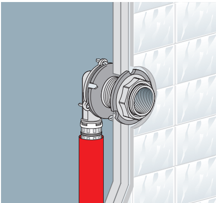
alpex hafif yapı duvar geçiş parçası
