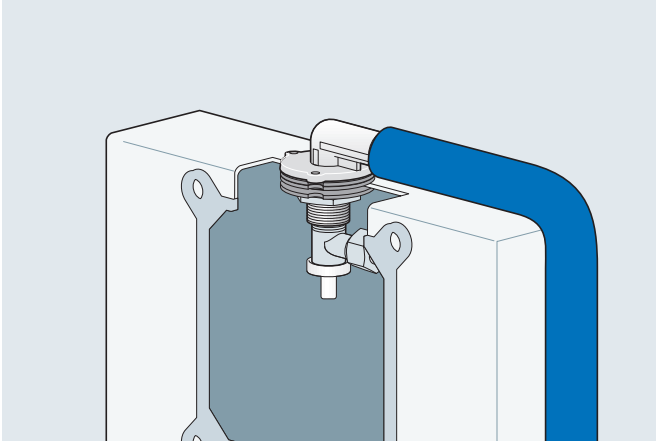
alpex SA rezervuar dirseği
