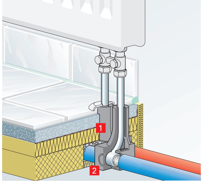
2 Ham zeminde ses köprüsünün engellenmesi
