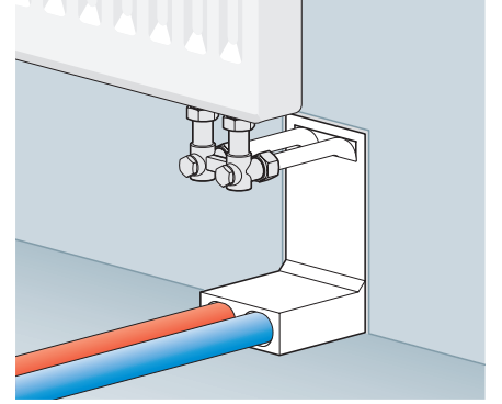
Radyatör bağlantı bloğuyla kolektörden alpex tekli bağlantı
