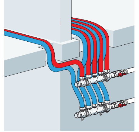
Bodrum kat tavanında kolektör montajı
