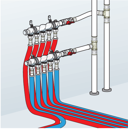
Bina kütlesinde kolektör montajı
