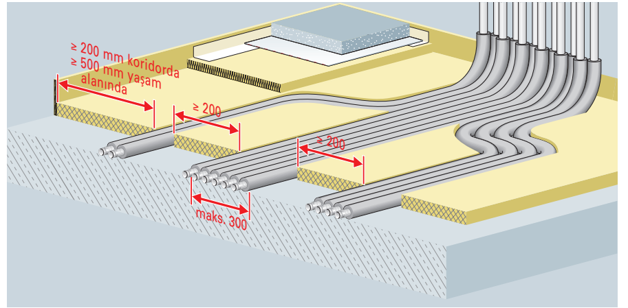
Boru demeti genişlikleriyle dayanma yüzeylerinin genişlikleri
