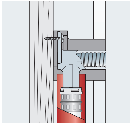
alpex duvar dirseği
