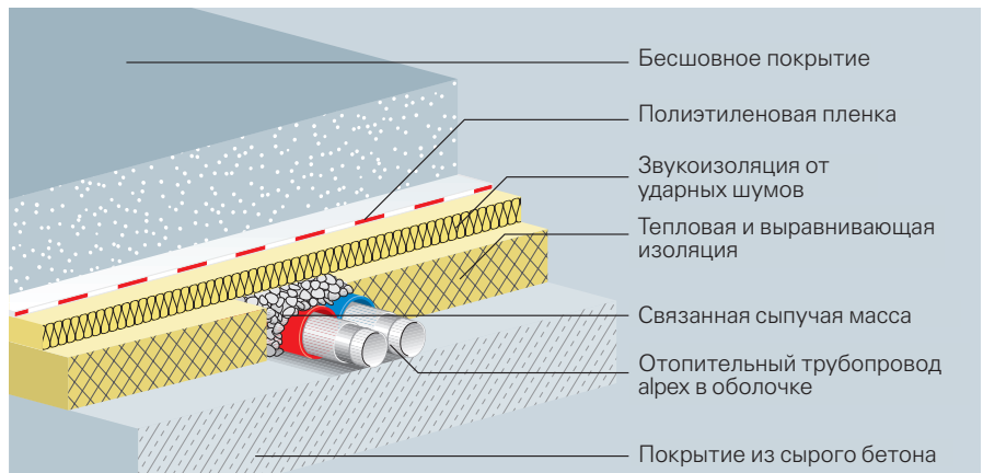
Конструкция пола под бесшовным покрытием с трубой alrex и надлежащей оболочке
