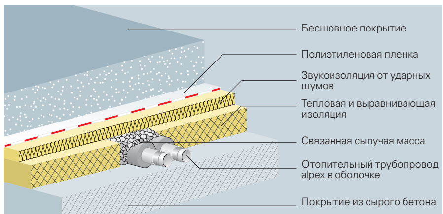
Конструкция пола под бесшовным покрытием с предварительно изолированной трубой alrex
