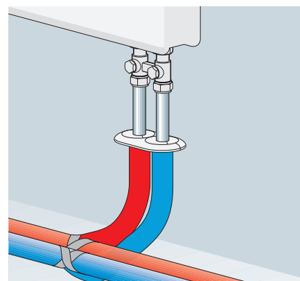
Тройниковая разводка alrex
